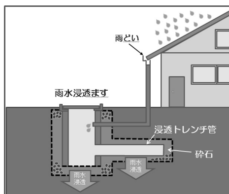
雨水浸透ます・トレンチ
